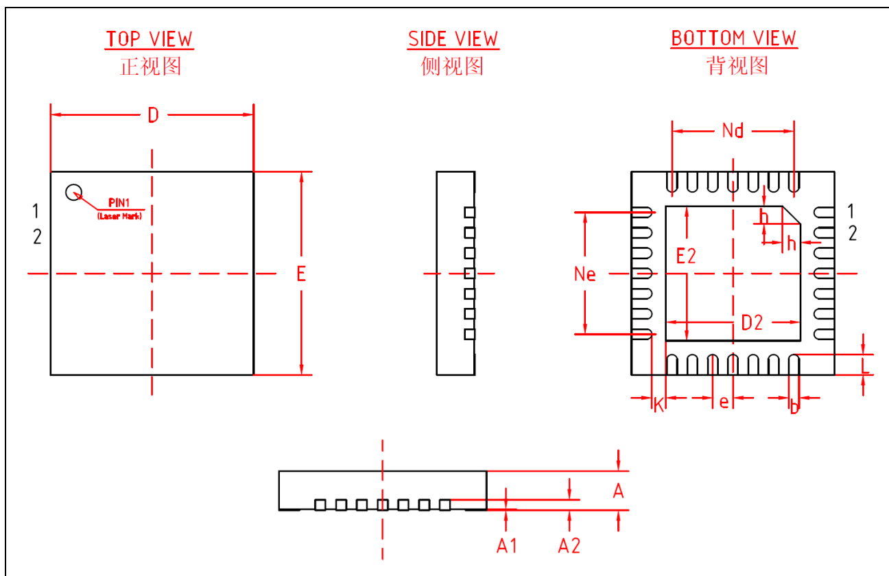
图 14-1 QFN28 封装图
